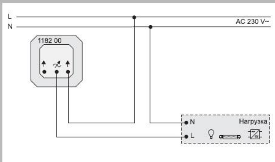
Подключение светорегулятора Троніс
